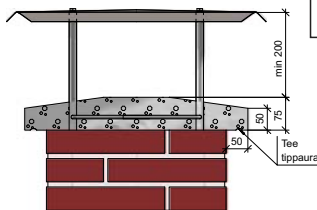
Poikkileikkaus
